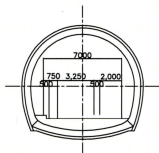
岸谷生麦線 (1方向部) J-J 断面
