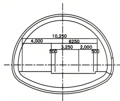
岸谷生麦線 (1方向部) I-I 断面
